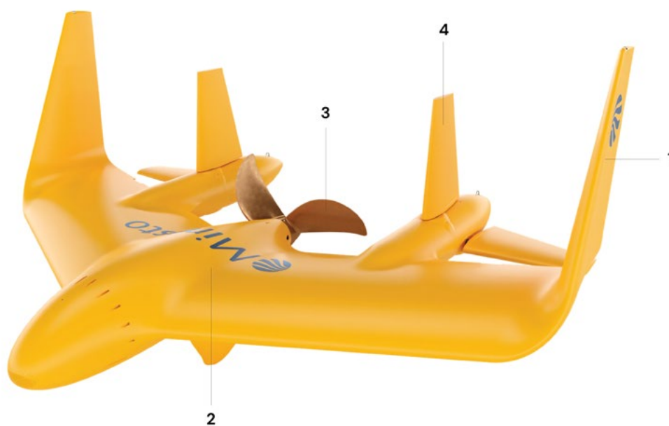
Bild 2. Minestos kraftverk består av en vinge (1) med ett maskinhus innehållande styrsystem och generator. (2) Bakom vingen sitter turbinen (3) och kraftverkets rodersystem. (4). Rodersystemet styr kraftverket automatiskt i en åttaformad bana. En förankringslina kopplar kraftverket till en bottenförankring i ett fundament på havsbotten. Förankringslinan rymmer elkablar såväl som kablar för kommunikation. Källa: Minesto
