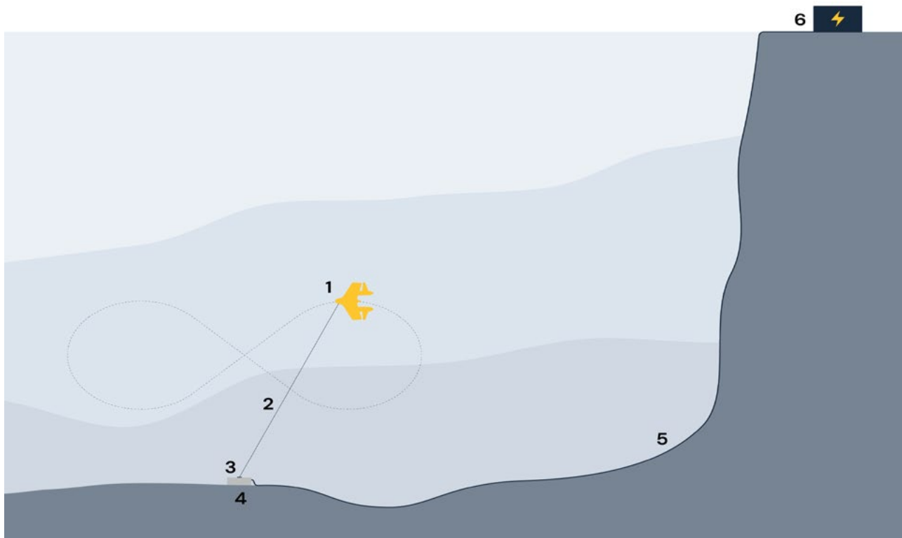
Bild 1. Illustration över de olika delarna vid en installationsplats för Minesto-teknik vilka är 1) Kraftverk som genererar elektricitet, 2) Förankringslina som kopplar ihop kraftverket med bottenförankringen, 3) Bottenförankringen som är kraftverkets rotationspunkt, 4) Fundament på havsbotten, 5) Sjökabel för kraftöverföring samt datakommunikation och 6) Anslutningspunkt till elnät. Källa: Minesto
